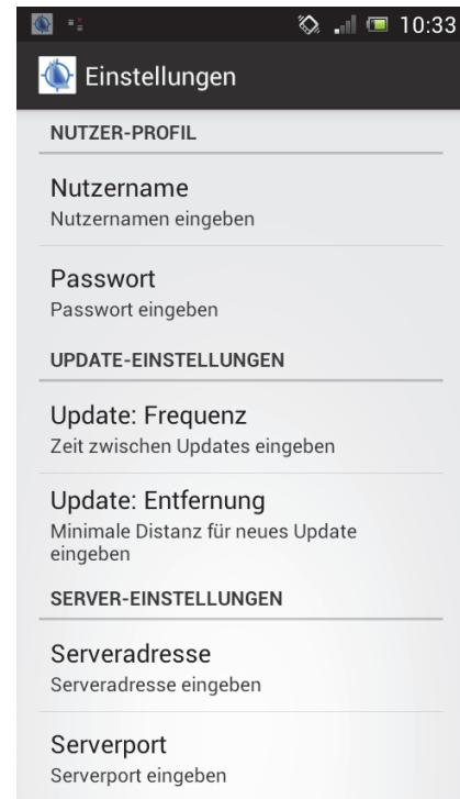
Abb. 2: Menü Einstellungen
